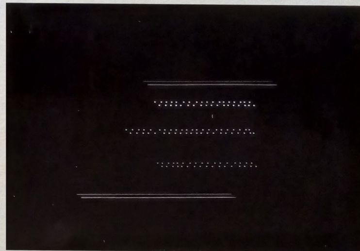
СНИМКИ ДВОЙНОЙ ЗВЕЗДЫ ГАММЫ ДЕВЫ
